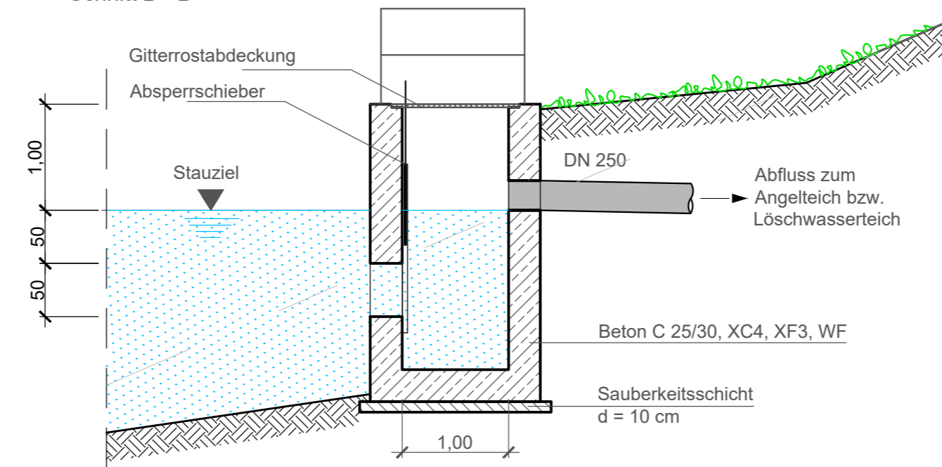
Schnitt B - B
